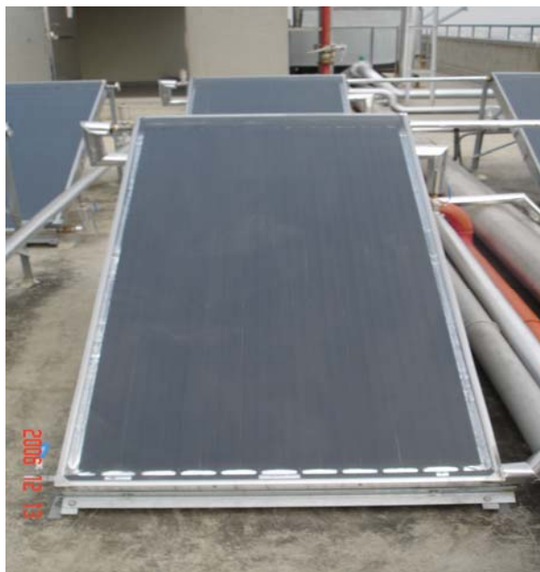
圖 6 宿舍太陽能系統設備
